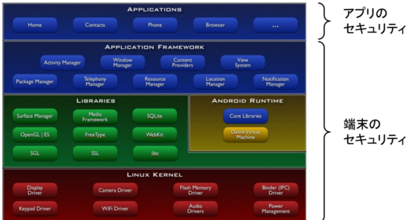
図 2.3.1 Android プラットフォームの主要コンポーネント
